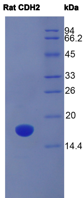
15% SDS-PAGE
