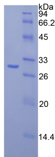
15% SDS-PAGE
