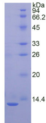
15% SDS-PAGE
