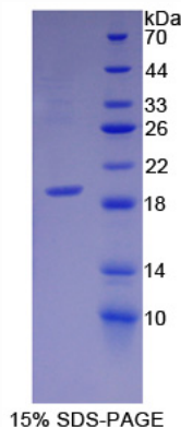
15% SDS-PAGE
