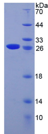
15% SDS-PAGE
