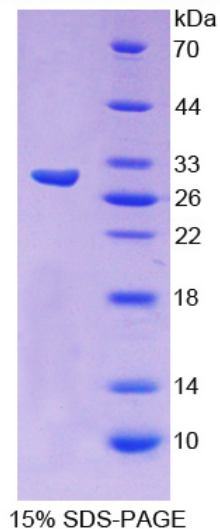
15% SDS-PAGE
