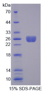
15% SDS-PAGE
